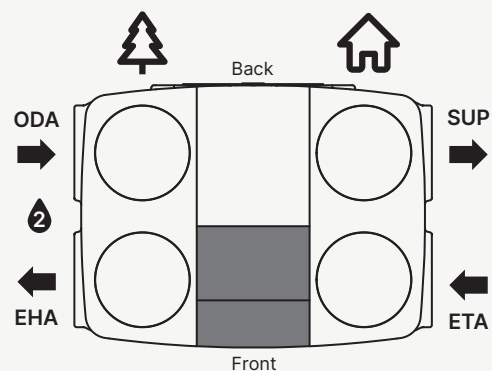
Rechtse positie
